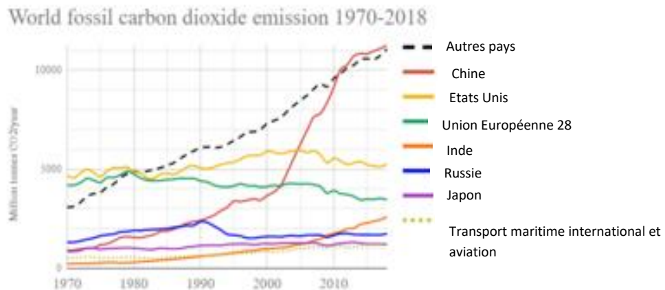
Figure N°2 : Le mode d'émission de CO 2 dans le monde dans la période 1970-2018
